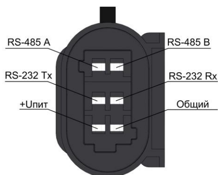
Рисунок 9. Разъем БИС 20240 для подключения внешнего устройства
