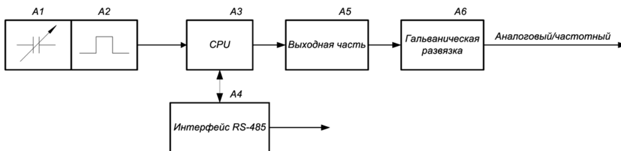
Рисунок 4. – Структурная схема изделия
